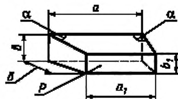
Рисунок 3 — Трапецидальный клин
